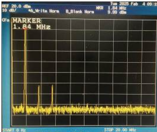
スプリアス領域（変調） 0-20MHz
