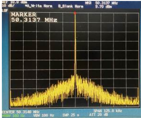
帯域外領域 (無変調)
