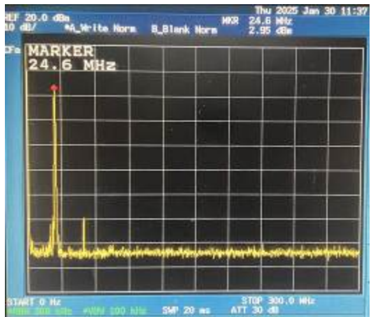
スプリアス領域 (変調) 0-300MHz
