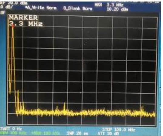
スプリアス領域（変調） 0-100MHz
