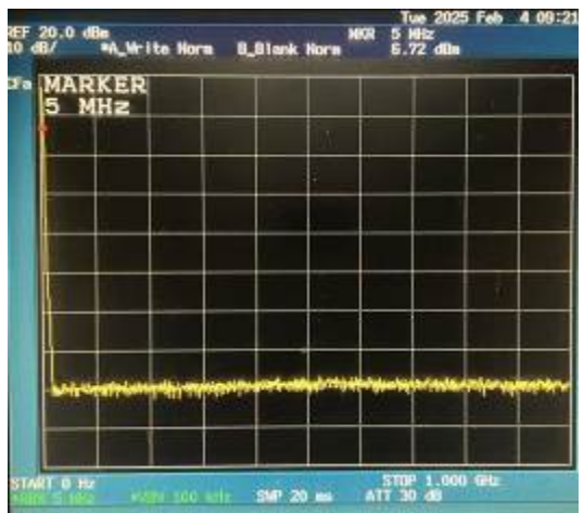
スプリアス領域（変調） 0-1GHz
