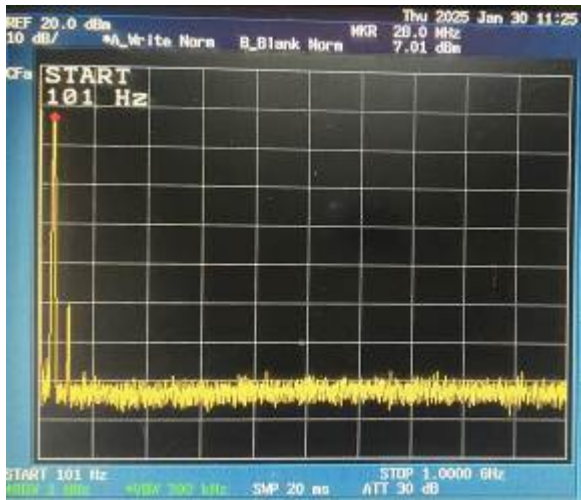
スプリアス領域 (変調) 0-1GHz
