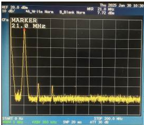
スプリアス領域 (変調) 0-200MHz
