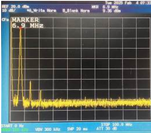
スプリアス領域 (変調) 0-100MHz
