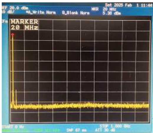
スプリアス領域 (変調) 0-1GHz
