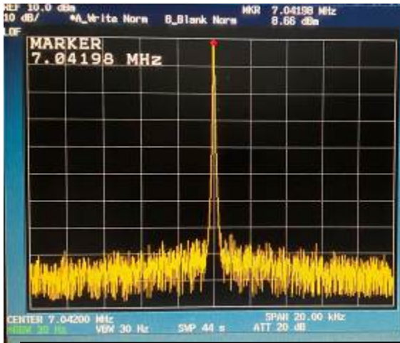
帯域外領域 (無変調)
