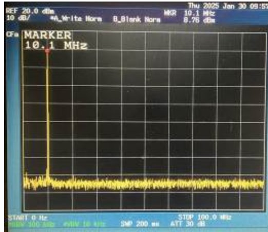
スプリアス領域 (変調) 0-100MHz
