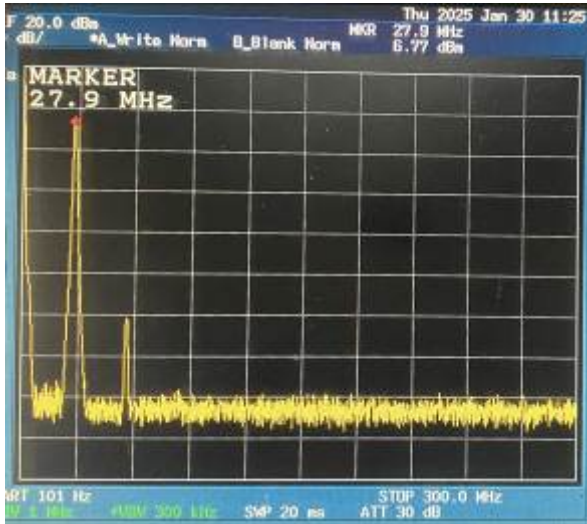
スプリアス領域 (変調) 0-300MHz
