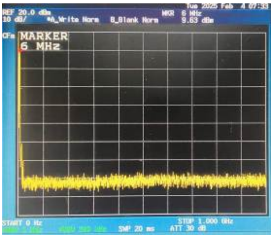
スプリアス領域 (変調) 0-1GHz
