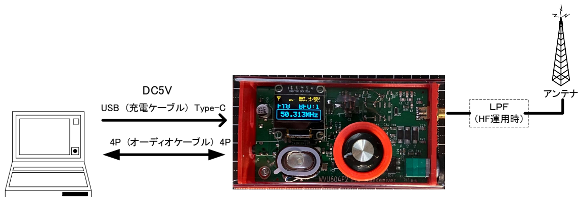
WVU604F2 接続図
